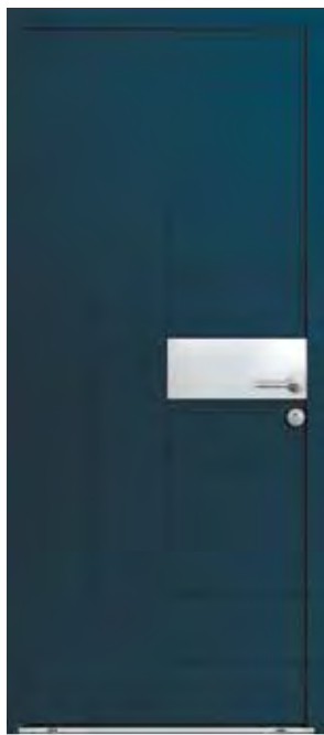
EXTÉRIEUR ALUMINIUM Couleur bleu 2700 sablé. Motif décor gravé. Insert décor aluminium brossé. INTÉRIEUR BOIS Finition pin cendré. Motif décor gravé. Ud \geq 0,7 \text{ W/m}^2\text{K}
