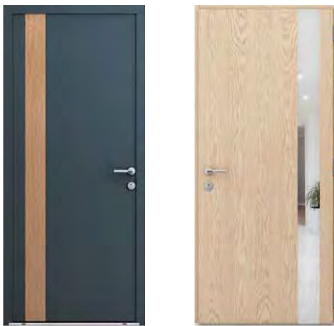
EXTÉRIEUR ALUMINIUM Couleur gris 7016 T. Insert décor ton bois. INTÉRIEUR BOIS Finition chêne champagne. Insert décor miroir. Ud ≥ 0,7 W/m².K
